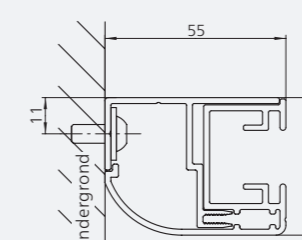
Kozijnmontage
